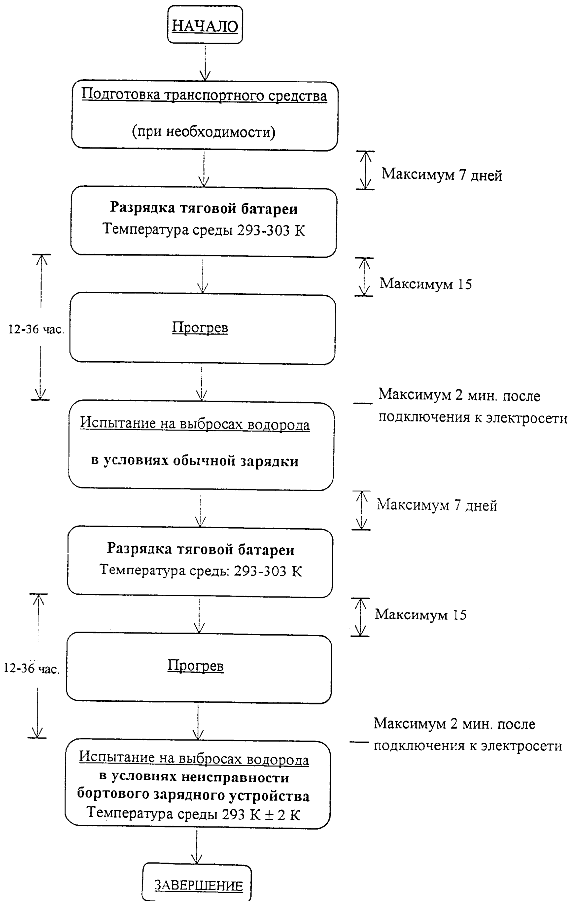
Рис. 7.1 Определение уровня выбросов водорода в процессе зарядки тяговой батареи
