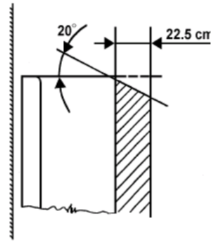
Longitudinal seat
