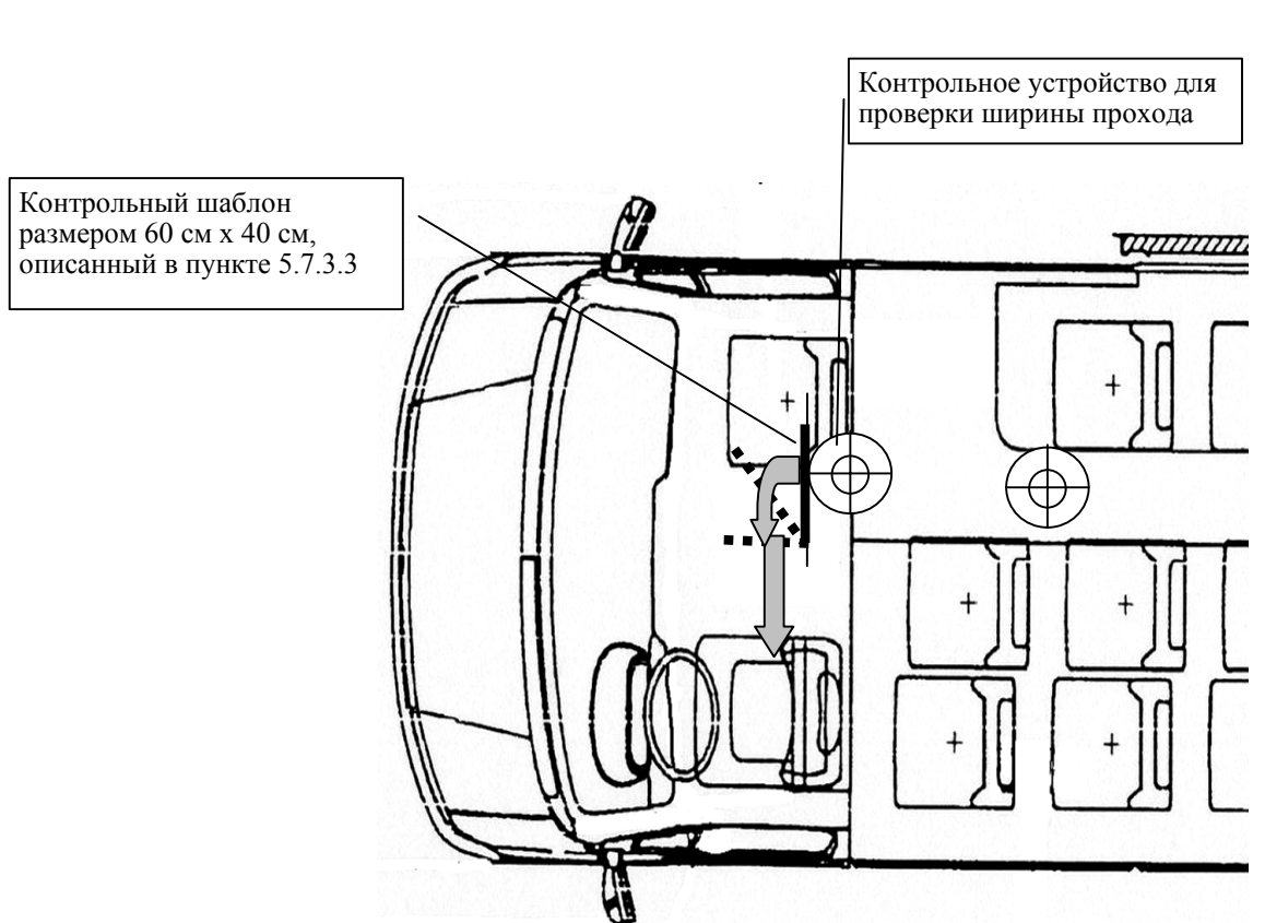
Рис. 22 ДОСТУП К ДВЕРИ ВОДИТЕЛЯ (См. пункт 5.7.2.4.2)
