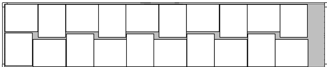
Figure 7.31 - Chargement d'unités de charge de 1 000 x 1 200 mm dans un conteneur de 40 pieds (12 m)
