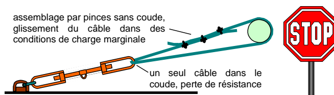
Figure 7.15 6 - Mauvais assemblage de saisine en câble métallique
