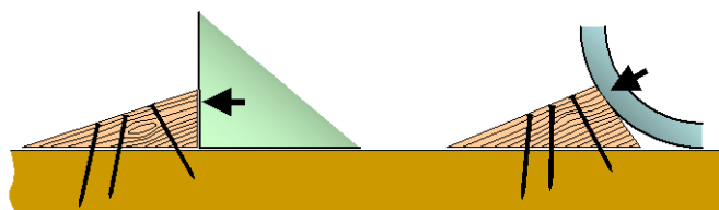
Figure 7.7 - Cales de blocage correctement taillées et clouées
