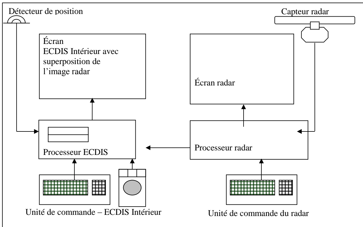
Appareil ECDIS Intérieur, système autonome relié à l'installation radar
