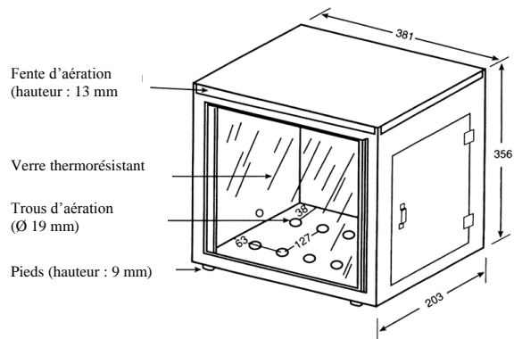
Figure 2 Toutes les dimensions sont en millimètres (mm)
