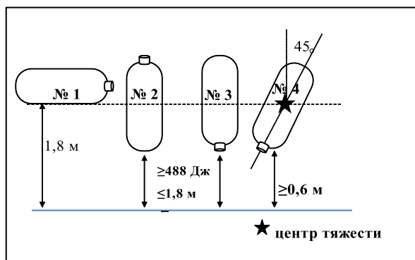
Рис. 1 Положения, в которых производят сбрасывание
