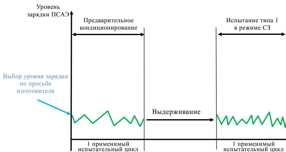
Рис. А8.Аpp1/5 ГЭМ-БЗУ и ГТСТЭ-БЗУ, испытание типа 1 в режиме сохранения заряда
