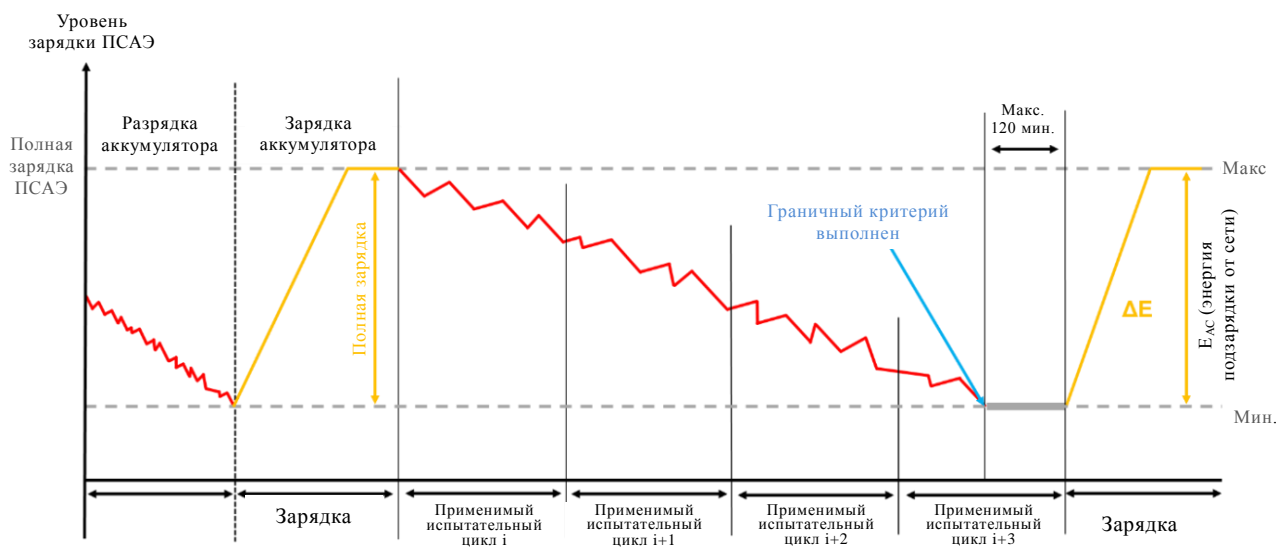
Рис. А8.Аpp1/6 Последовательность испытания ПЭМ с прогнозом по последовательным циклам
