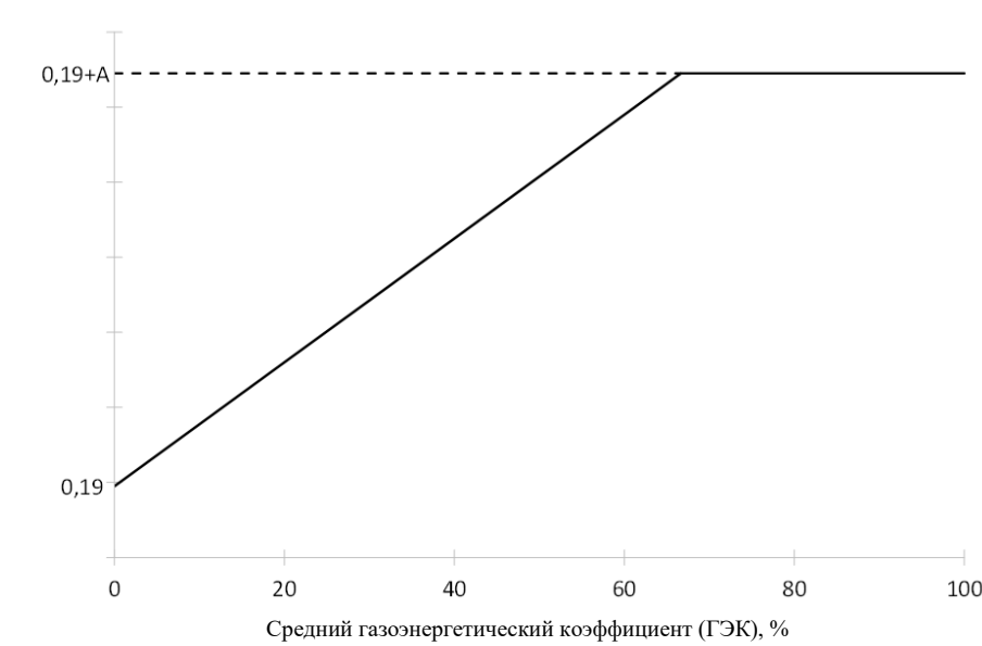
График зависимости предельного значения выбросов НС от среднего ГЭК
