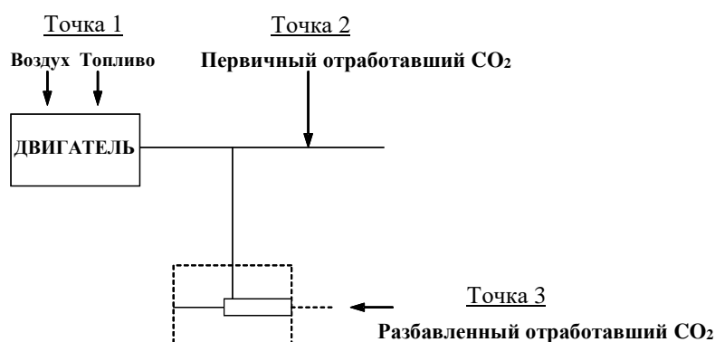
Система частичного разбавления потока
