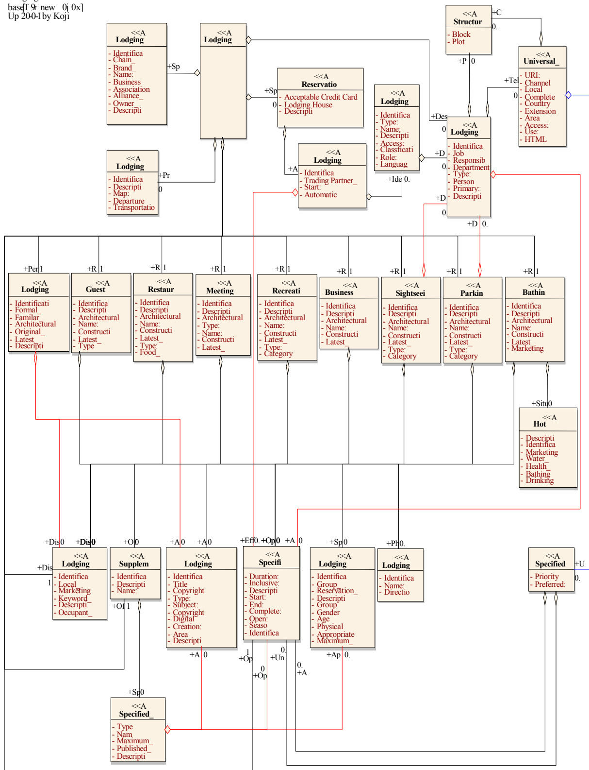
Рисунок 3. Диаграмма классов: информация о пансионатах
